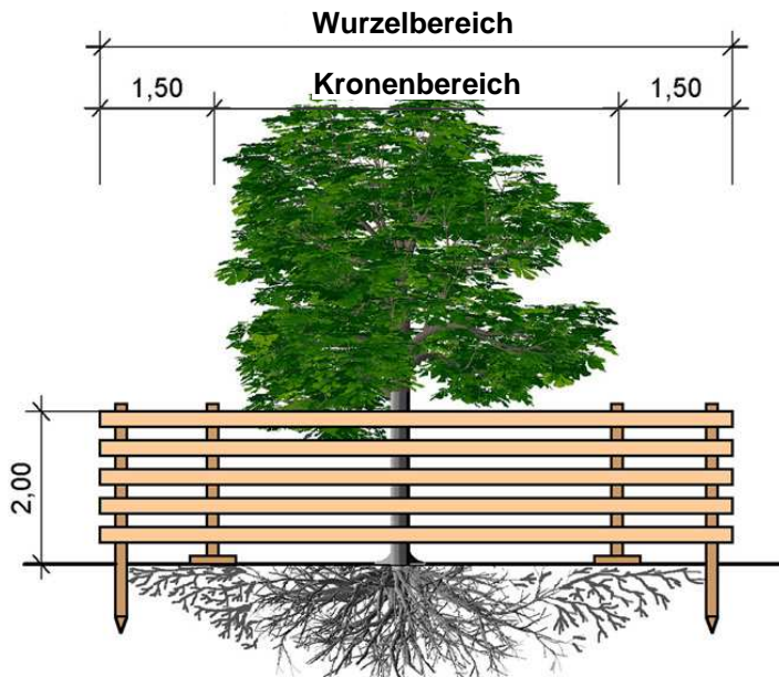
Standardlösung: Wurzelschutz durch einen ortsfesten Zaun
