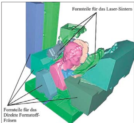
Die Formteile für das Laser-Sintern
